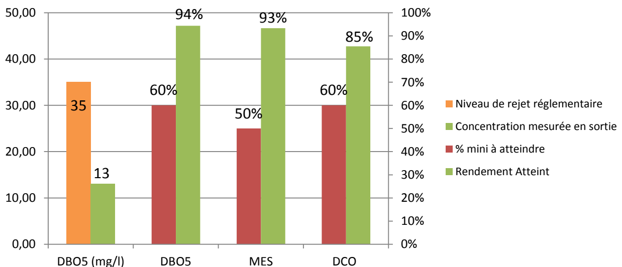
Sortie STEU Saint Bardoux Village : performances épuratoires
